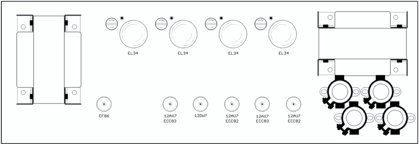
Röhrenbestückung Spectro 100 Serie
