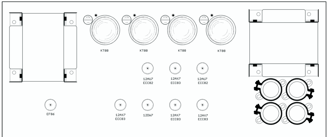
Röhrenbestückung Spectro 200 Serie mit aktiver Klangregelung
